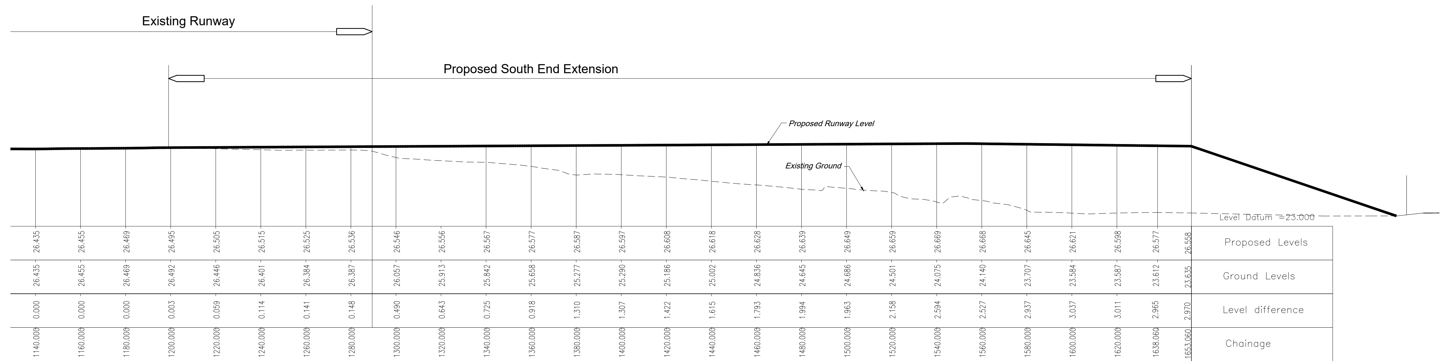
LONGITUDINAL SECTION
